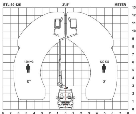
Bočný dosah so zaťažením koša 120 kg 0°
