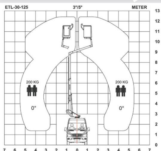
Bočný dosah so zaťažením koša 200 kg 0°
