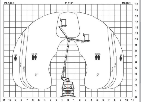
Bočný dosah so zaťažením koša 120 / 200 / 230 / 265 kg 0°
