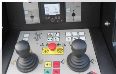
Proporcionálne CANbus ovládanie s displejom
